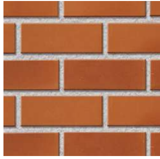
Cintilla de Barro 2VC 24x6x1.5 cm 57 Pzas/m 2 .4kg/pza
