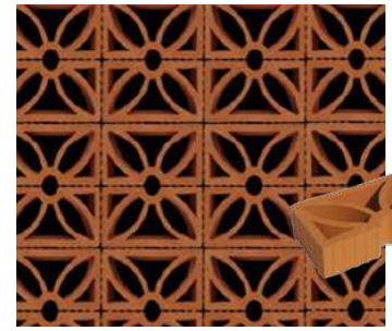
Celosía N° 5 1.6kg/pza 30 pzas/m 2 • 24x13x6cm
